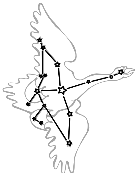
Cygnus
