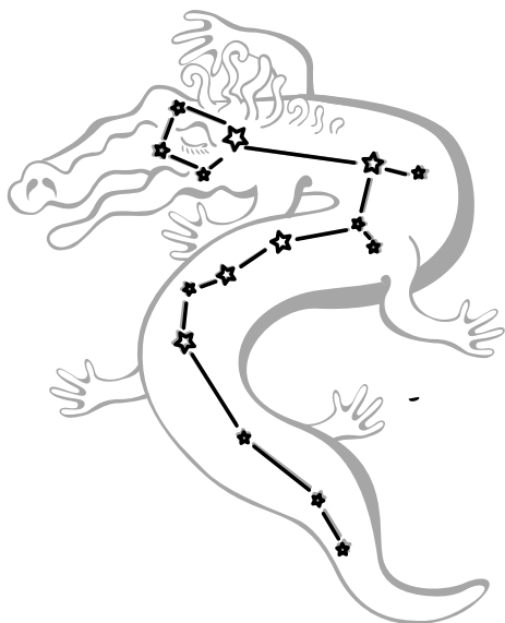
Draco
