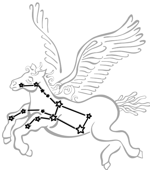
Pegasus
