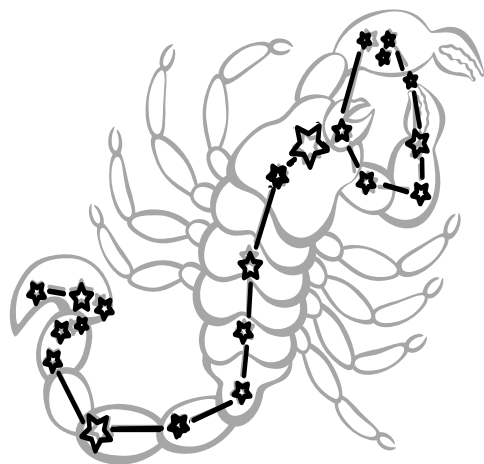
Scorpio
