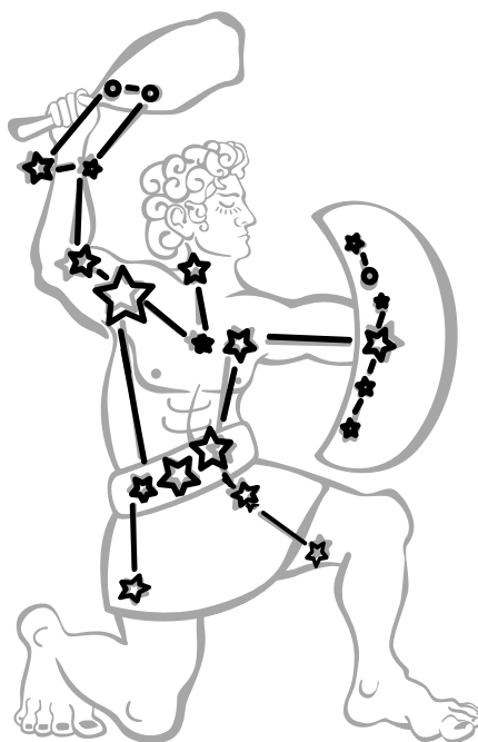
Orion
